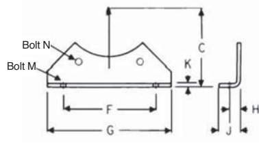
Flange Foot
